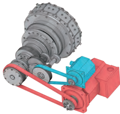
铣刀马达使用主轴马达驱动，换刀马达使用伺服马达驱动。
