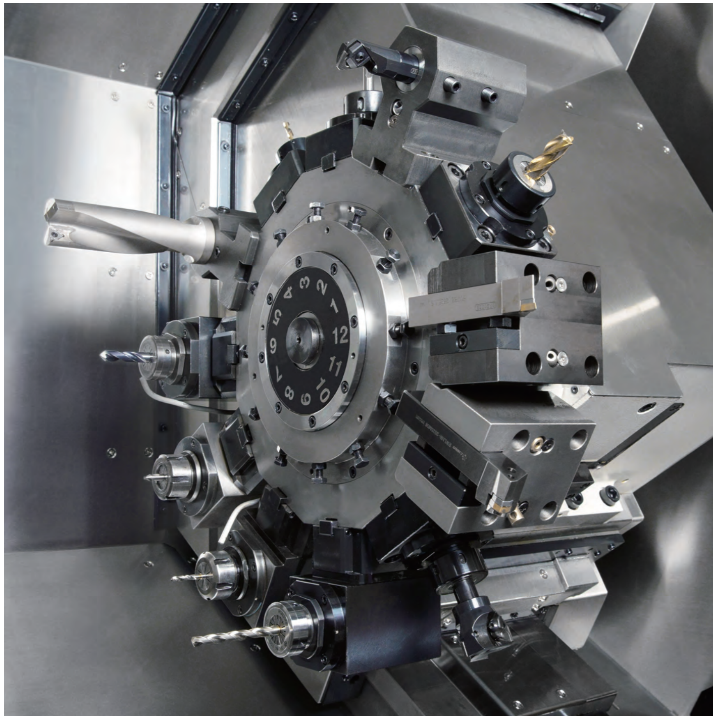
铣刀马达使用主轴马达驱动，换刀马达使用伺服马达驱动。
